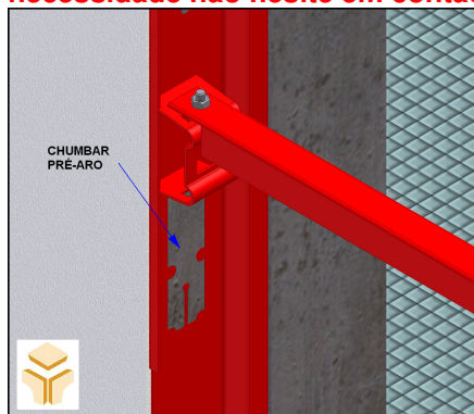
Fig. 1.8 – Chumbar pré-aro
