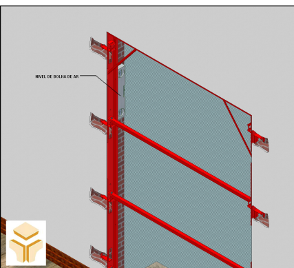
Fig.1.7 – Assentar e nivelar o pré-aro
