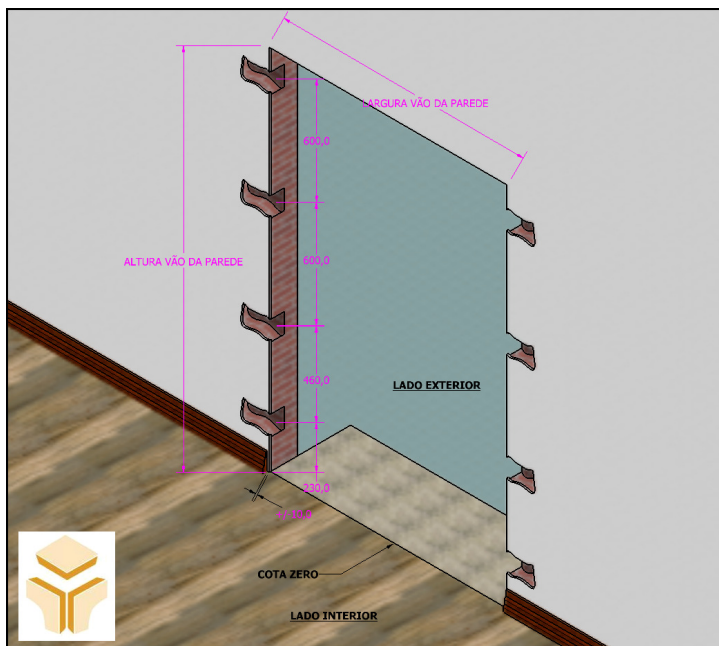
Fig.1.4 – Abertura de rasgos para introdução do pré-aro
