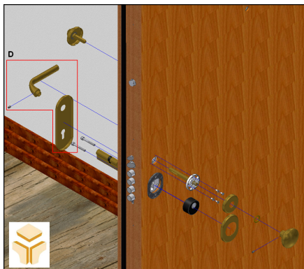
Fig. 3.6 – Montagem de ferragens (D)
