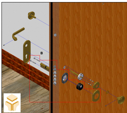
Fig. 3.4 – Montagem de ferragens (B)
