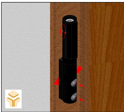
Fig. 3.2 – Regulação da porta em altura largura da folha
