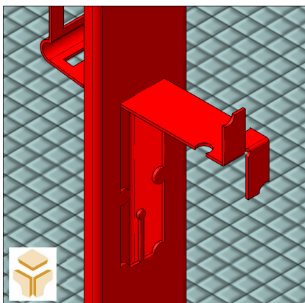
Fig. 1.5.2 – Garra preparada
