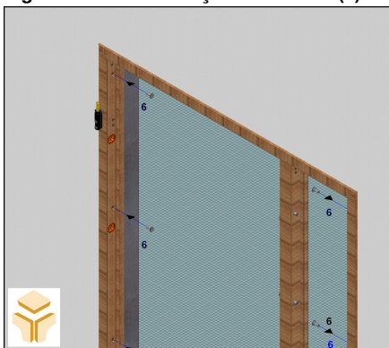
Fig.2.2 – Colocação dos parafusos de aperto do aro ao pré-aro
