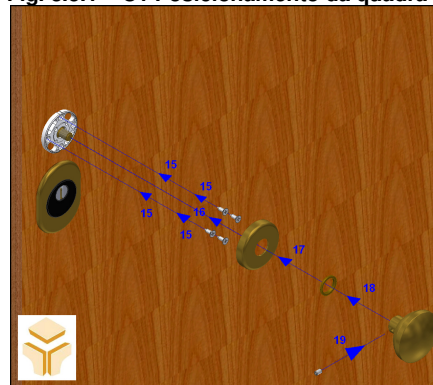
Fig. 3.5.3 – C3 Colocação base, espelho da bola e bola (15) (16) (17) (18) e (19)
