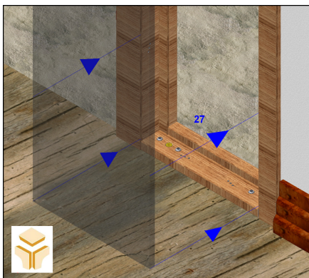
Fig. 4.1 – Instalação do vidro
