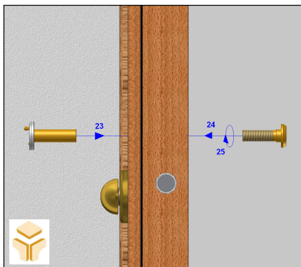
Fig. 3.7.1 – E1 Colocação do óculo
