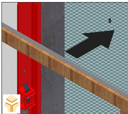
Fig.2.1.2 – D2 Assentamento do pré-aro (5)
