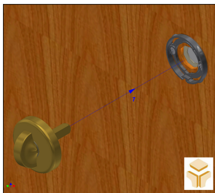
Fig. 3.3 – Montagem do espelho e manipulo do limitador de abertura (A)
