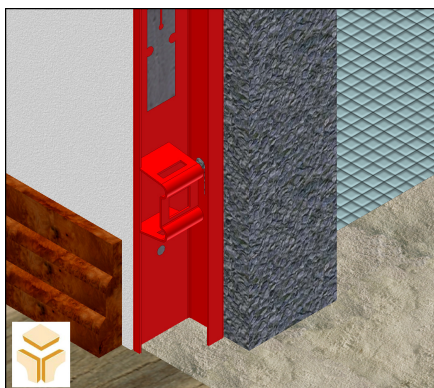
Fig.1.2 – Acabamento em cantaria de pedra
