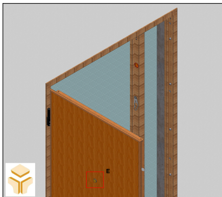
Fig. 3.7 – Montagem de ferragens (E)
