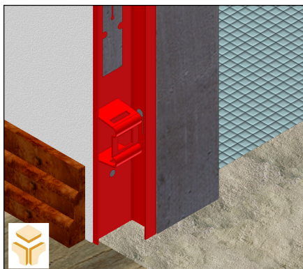
Fig.1.1 – Acabamento com reboco
