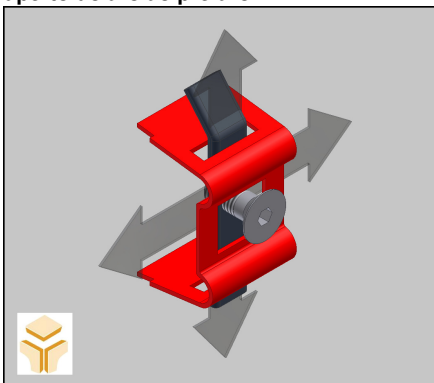
Fig. 2.3 – Pré-ajustamento (jogo de movimentos: conjunto estafa-parafuso-aro)
