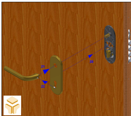
Fig. 3.6.1 – D1 Colocação e aperto do
