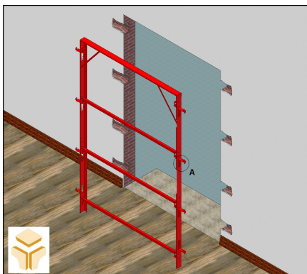
Fig. 1.5 – Dobrar garras do pré-aro (A)
